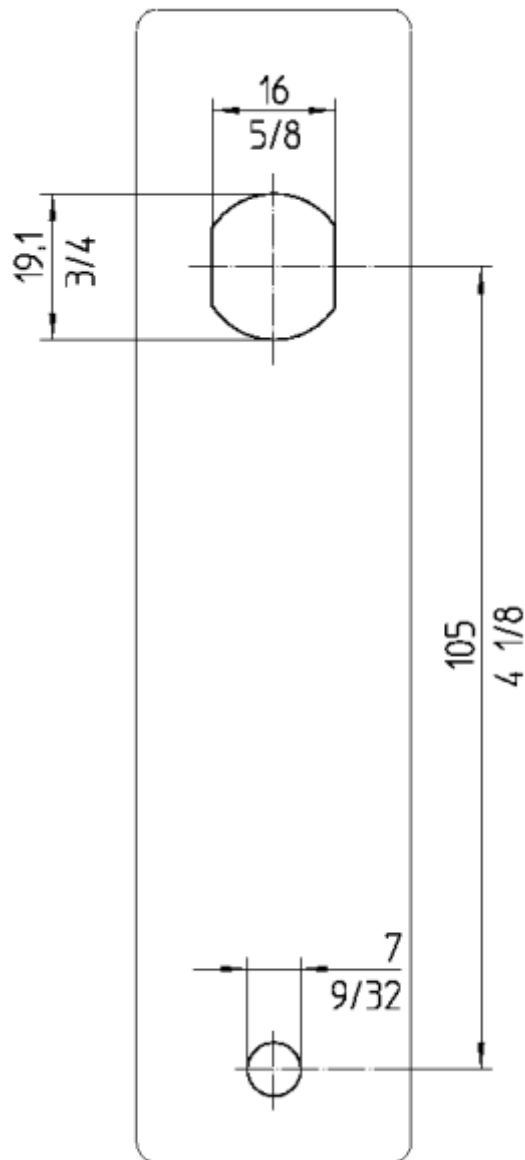
Abbildung 9.2 – Bohrschablone
