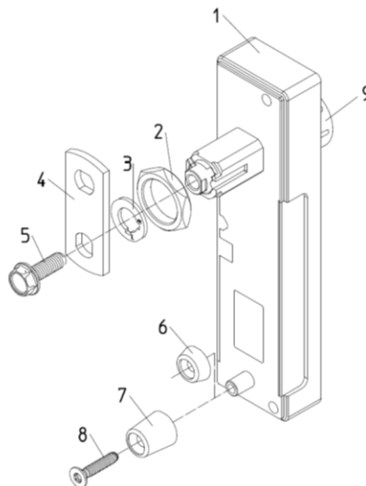
Abbildung 2.1 – Montage des Schlosses
