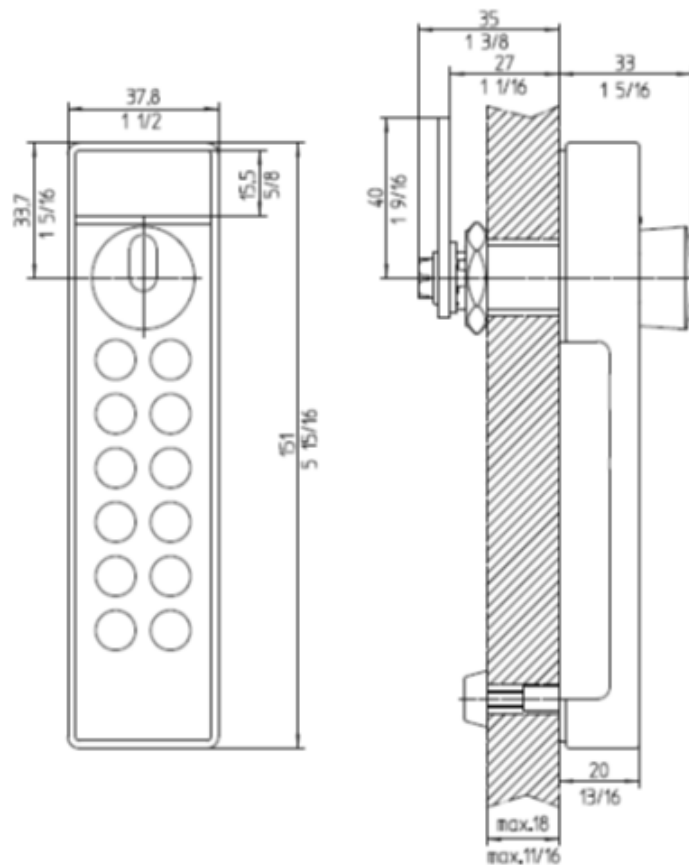
Abbildung 9.1 – Technische Abmaße
